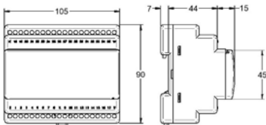
6 Moduli DIN - LCD display
