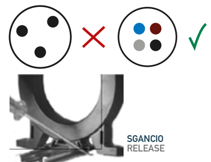
PASSAGGIO CAVI CORRETTO CORRECT CABLES PASSAGE
